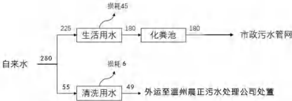
图2-3 水平衡图（单位t/a）
