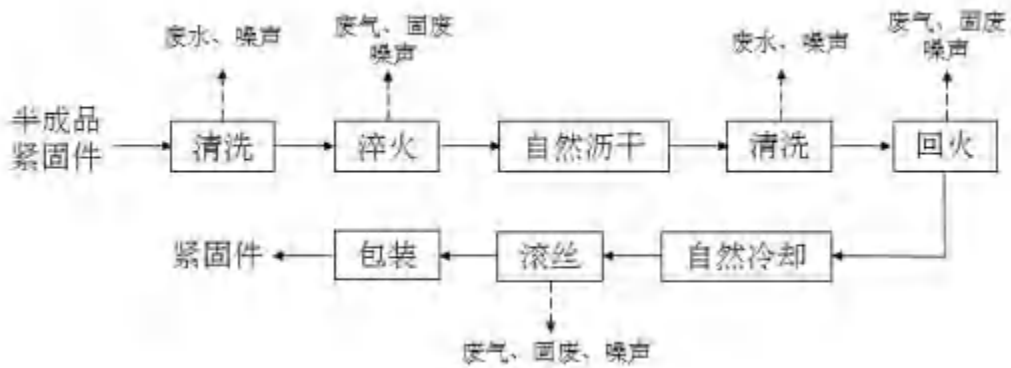
图2-4 生产工艺及产污流程图
