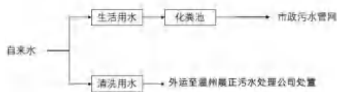
图3-1 废水排放去向图
