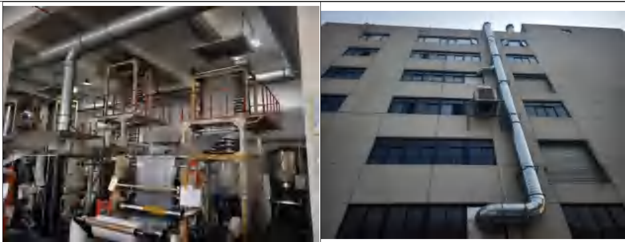
吹膜、印刷废气集气照片
