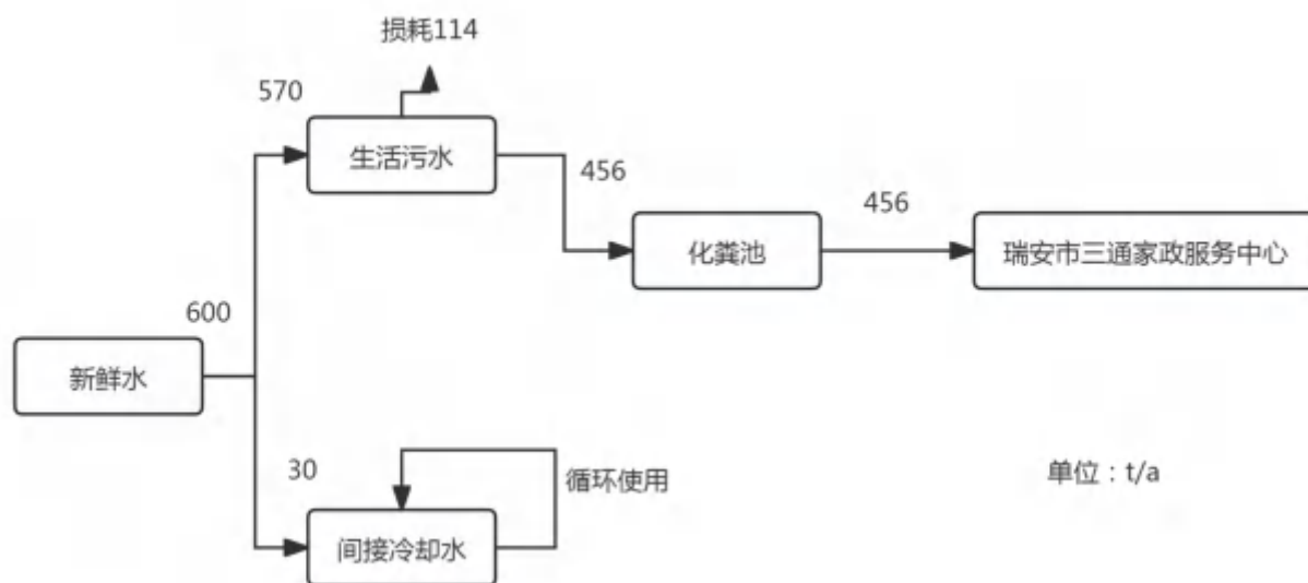
图2-3 水平衡图
