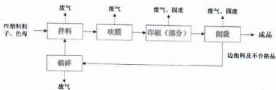
塑料薄膜袋生产工艺流程及产污环节示意图
