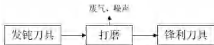
图2-5 刀具修理工艺及产污流程图
