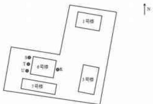
● S、T、U、E—无组织废气采样点
