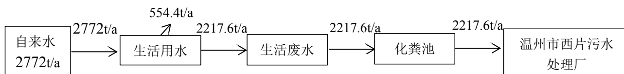
图2-3 水平衡图
