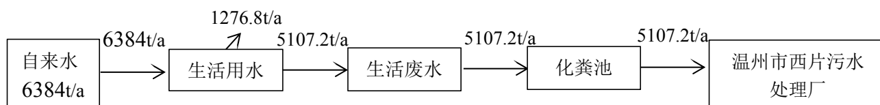
图2-3 水平衡图
