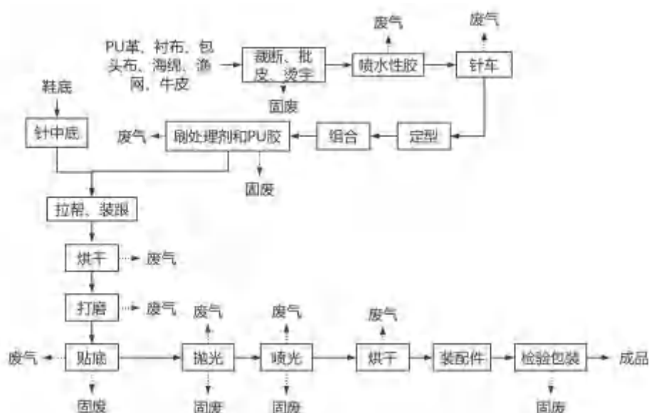
图2-4 女鞋生产工艺流程及产污环节示意图
