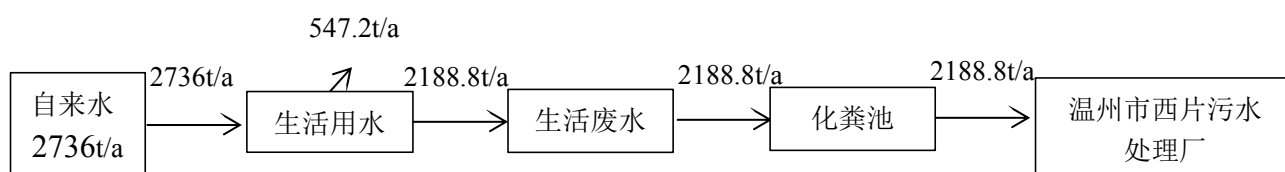
图2-3 水平衡图
