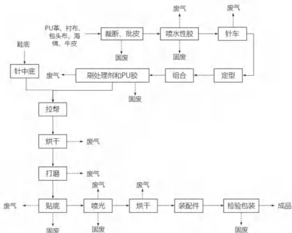
图2-4 女鞋生产工艺流程及产污环节示意图
