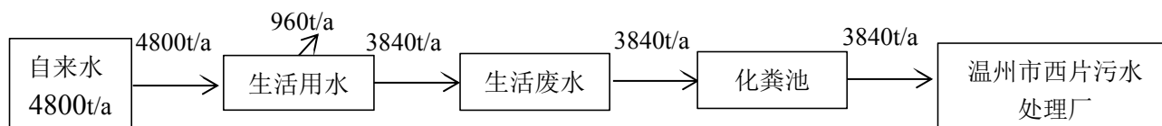
图2-3 水平衡图
