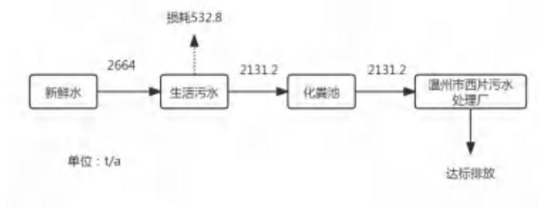
图2-3 水平衡图
