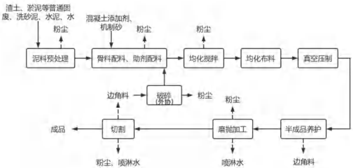
图2-5 生产工艺流程及产污环节示意图
