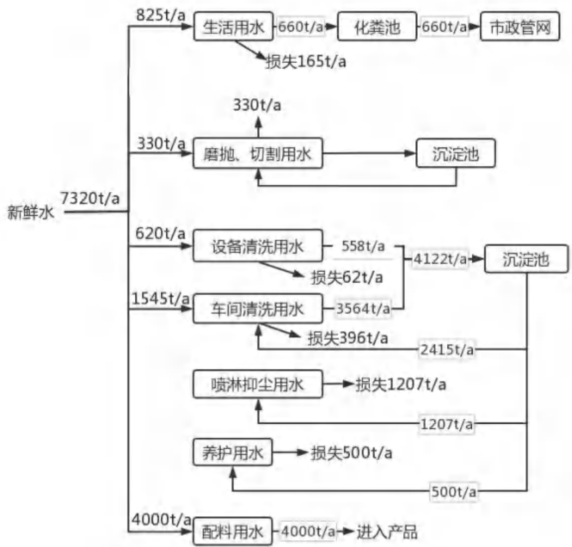
图2-4 水平衡图
