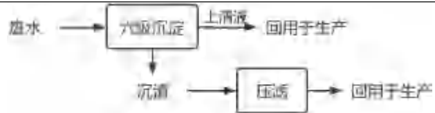
图3-2 生产废水处理工艺流程
