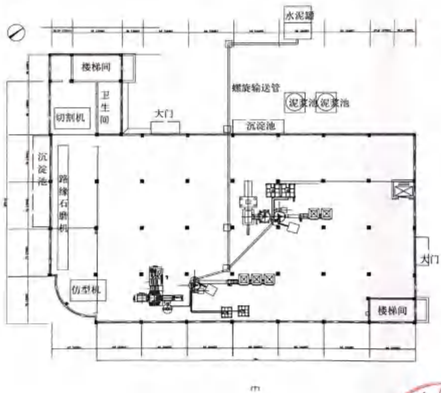
车间平面图
