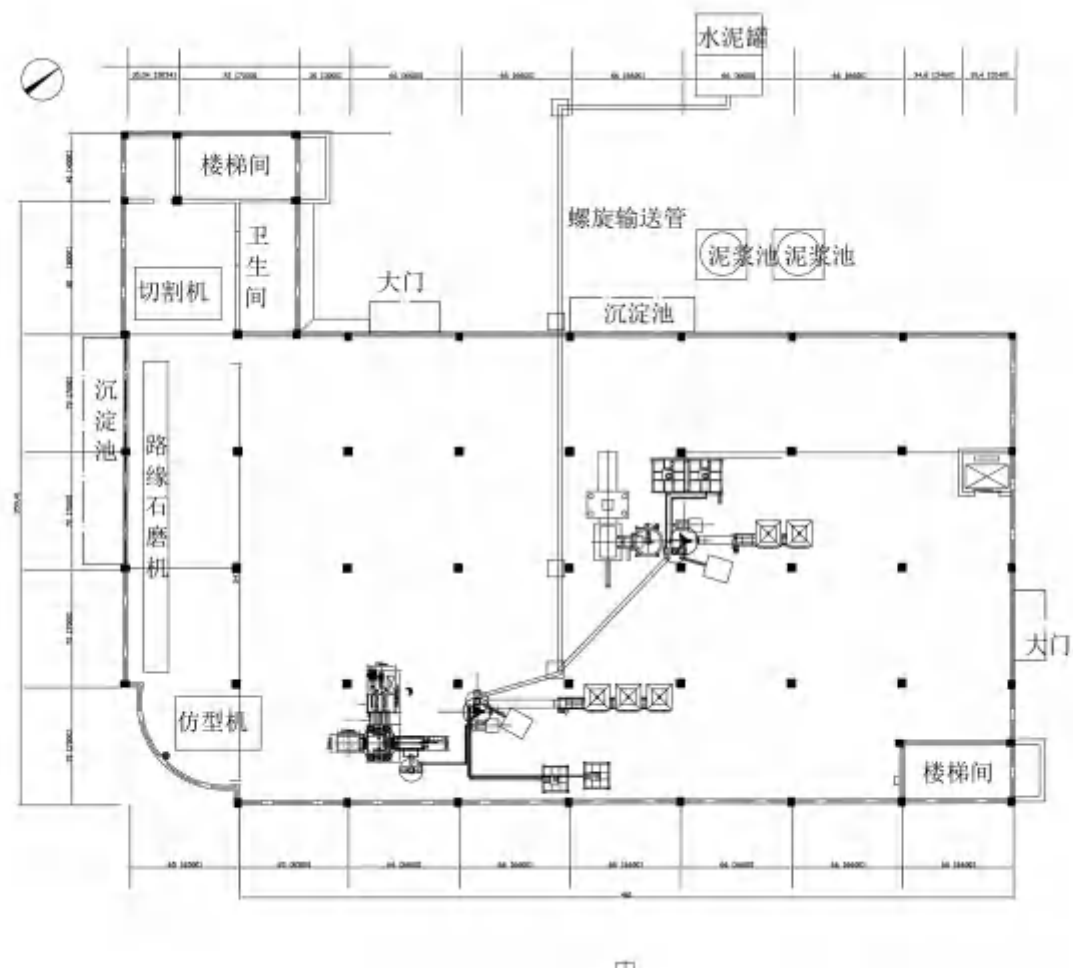
图2-3 车间平面图
