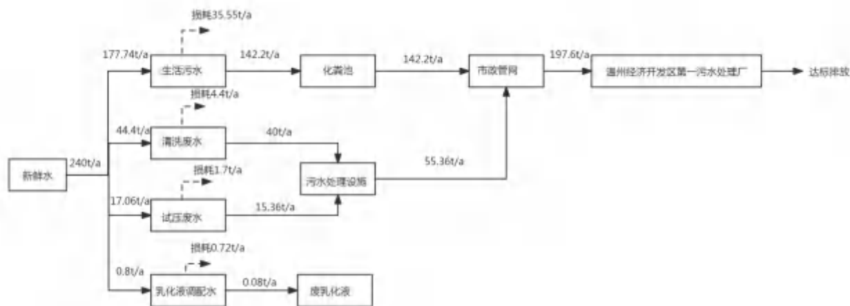
图2-3 水平衡图
