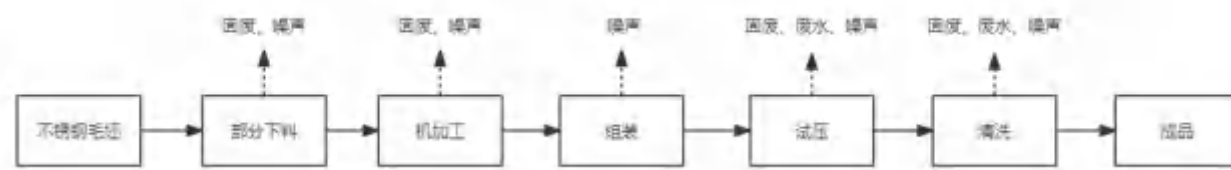
图2-4 阀门生产工艺流程及产污环节示意图
