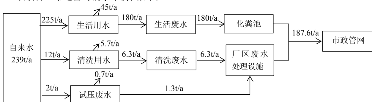
图2-3 水平衡图
