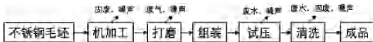
图2-4 项目生产工艺及产污环节示意图
