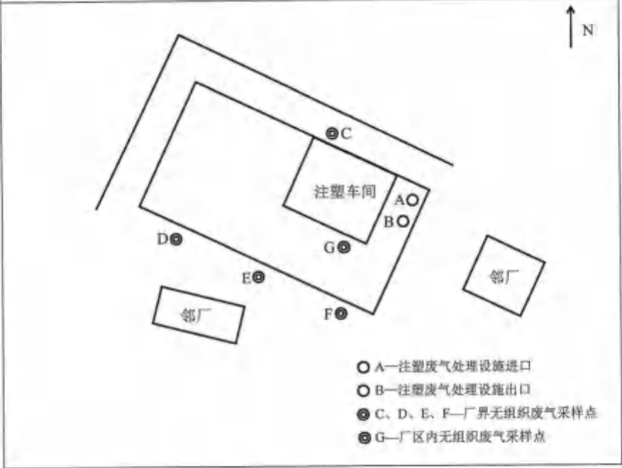
废气采样点位示意图
