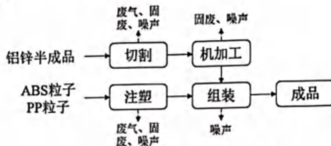
图 2-2 门锁配件生产工艺及产污流程图
