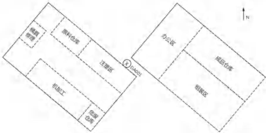
图2-2 厂区平面图
