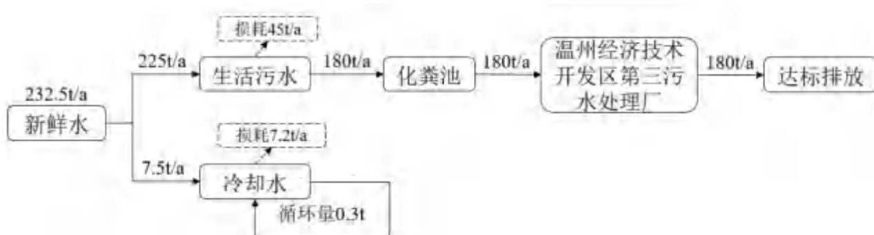
图2-3 水平衡图
