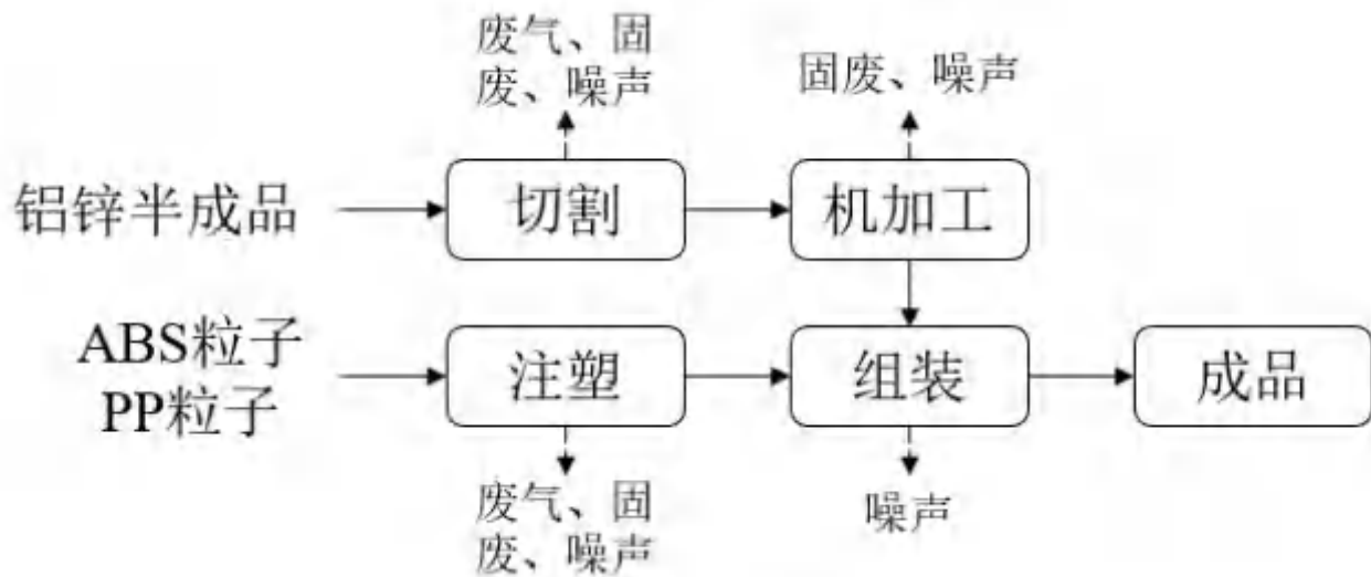
图2-4 门锁配件生产工艺及产污流程图
