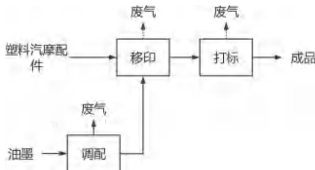
图2-3 生产工艺及产污流程图
