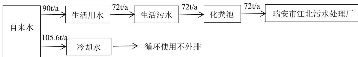
图2-4 水平衡图
