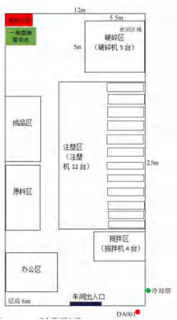
图2-2 厂区平面图
