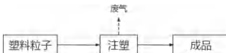
图2-3 生产工艺及产污流程图
