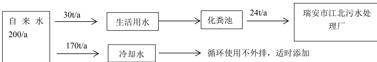
图2-4 水平衡图
