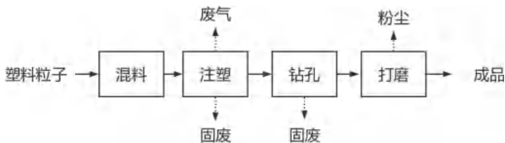
图2-3 生产工艺及产污流程图
