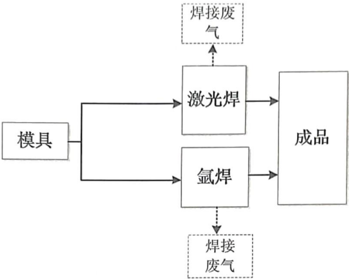
图2-2 生产工艺流程图
