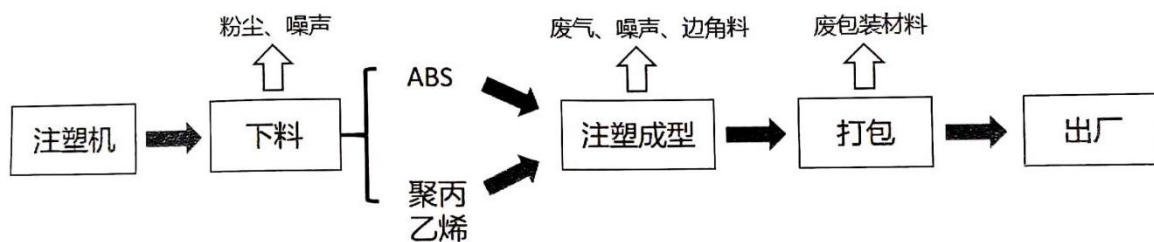
图2-2 项目生产工艺及产污环节示意图
