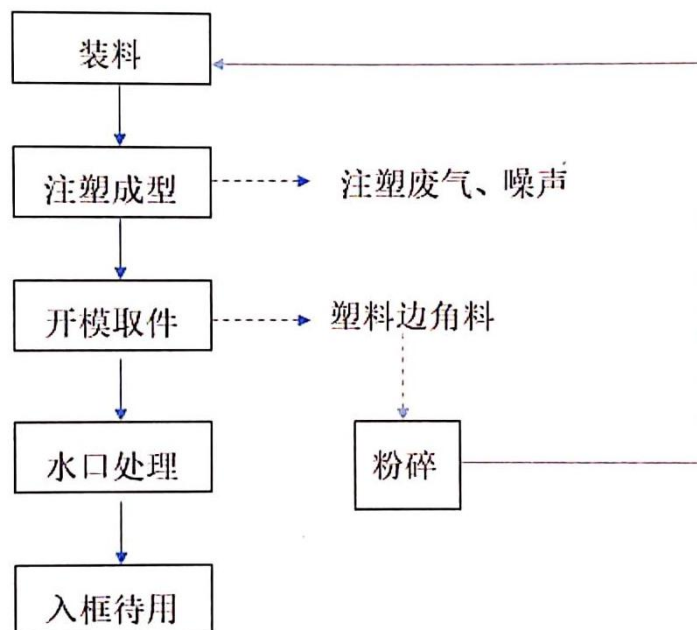
图2-2 项目生产工艺及产污环节示意图
