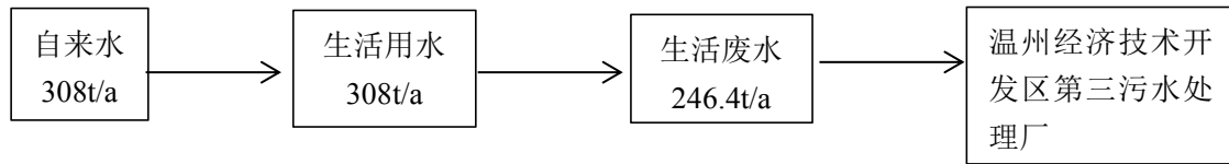
图2-2 水平衡图
