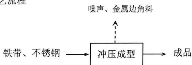
锁配件工艺流程
