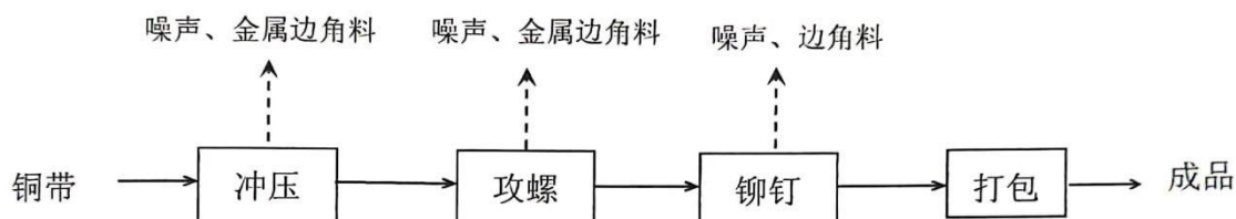
电器配件工艺流程
