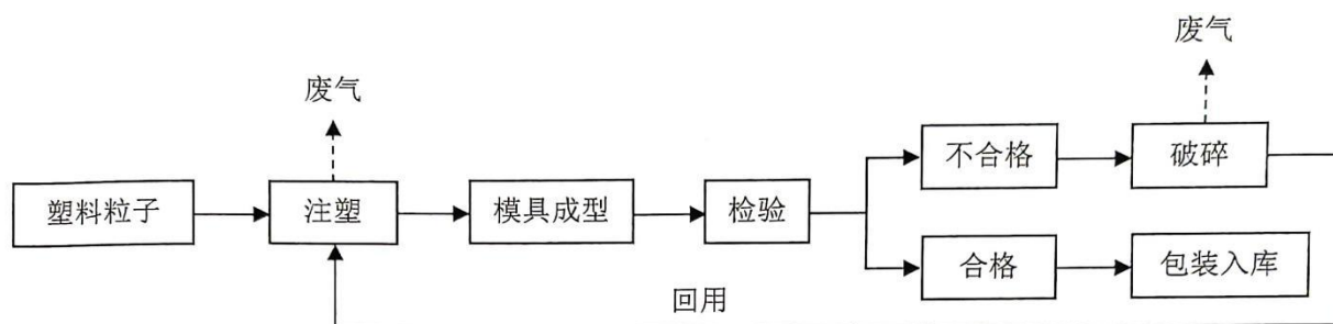
图2-2 项目生产工艺及产污环节示意图
