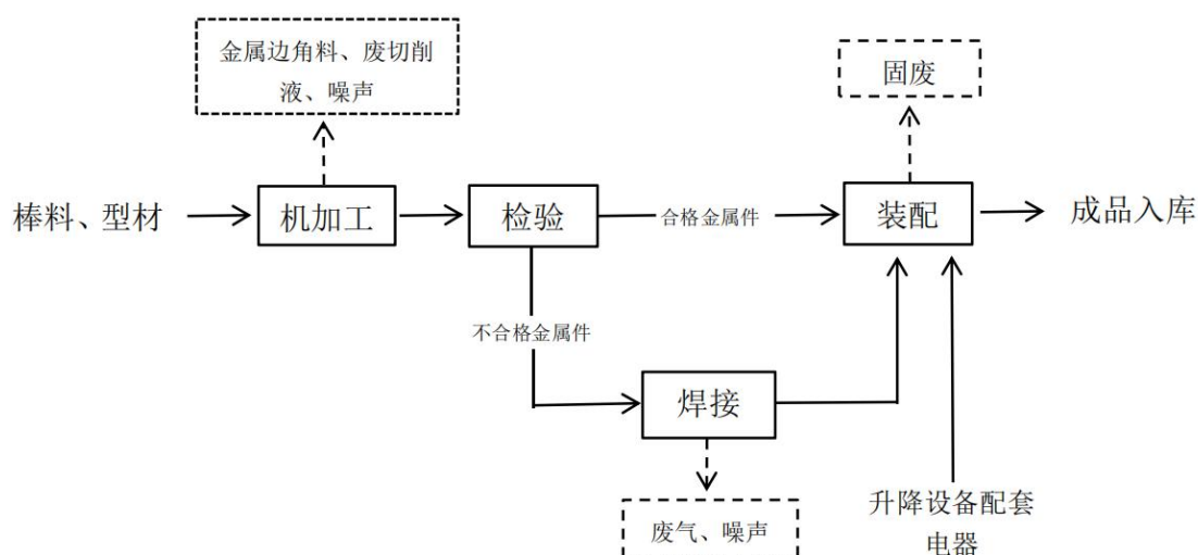
图2-4 升降设备工艺流程图
