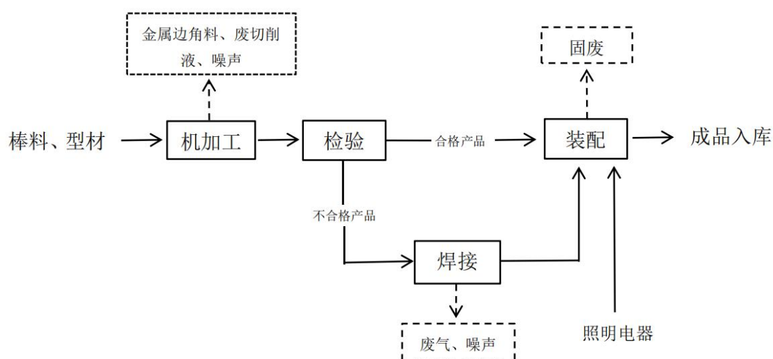
图2-3 照明设备工艺流程图
