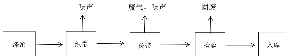
图2-3 项目生产工艺及产污环节示意图
