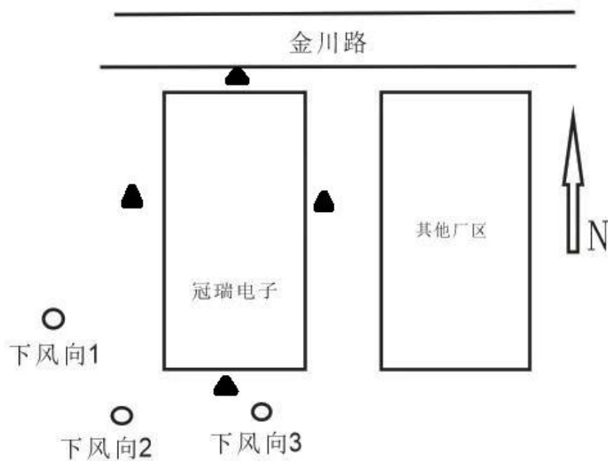
图6-1 废气、噪声监测点位图
