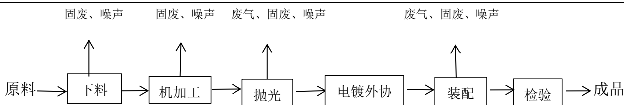
图2-3 项目生产工艺及产污环节示意图
