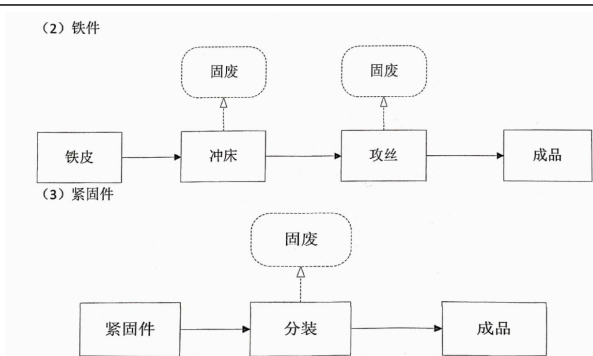
图2-3 项目生产工艺及产污环节示意图
