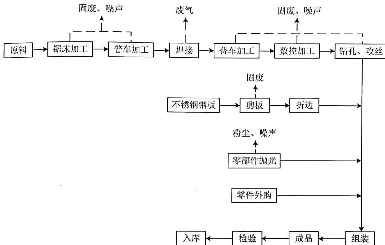
图2-2 项目生产工艺及产污环节示意图
