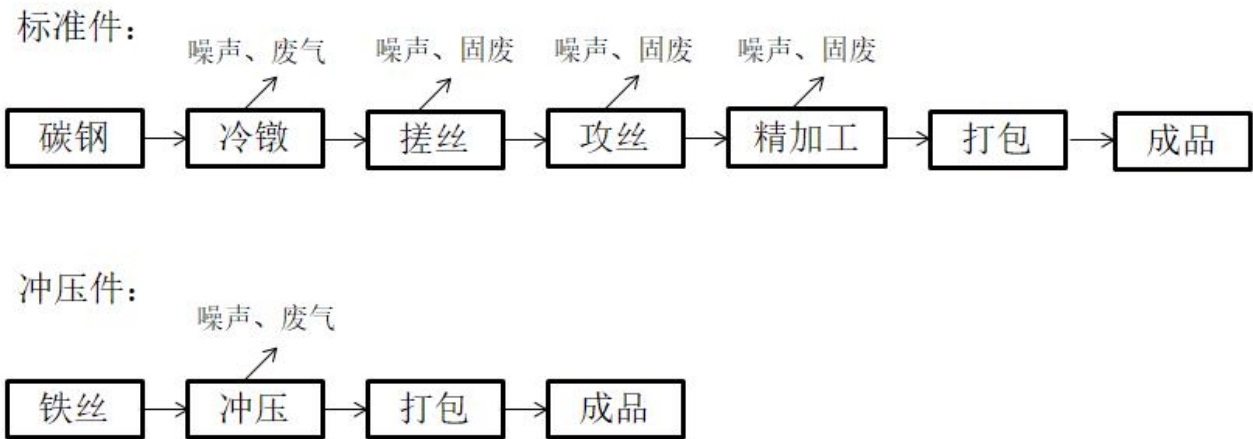
图2-2 项目生产工艺及产污环节示意图
